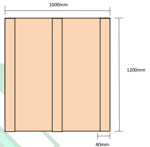
Vista Inferior
