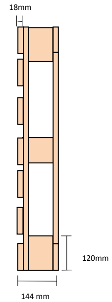
Vista Lateral
