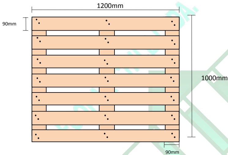
Vista Frente
